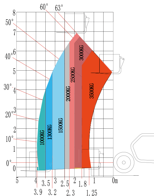
CURVA DE CARGA DEL H735 EN CONDICIONES RT
